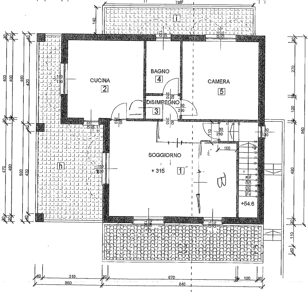
PIANTA PIANO PRIMO 1:100
