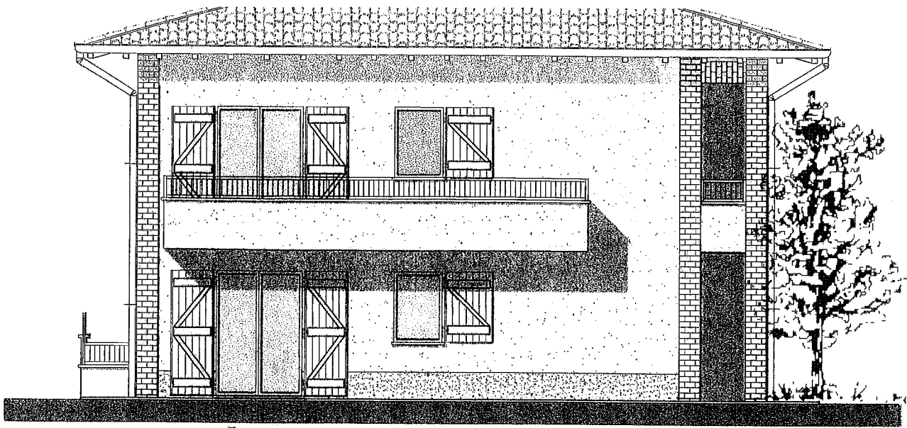
PROSPETTO NORD 1:100
