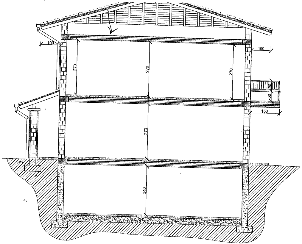
SEZIONE A-A 1:100
