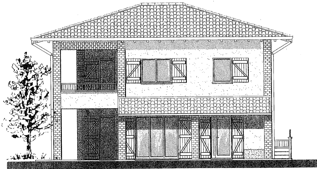
PROSPETTO SUD 1:100
