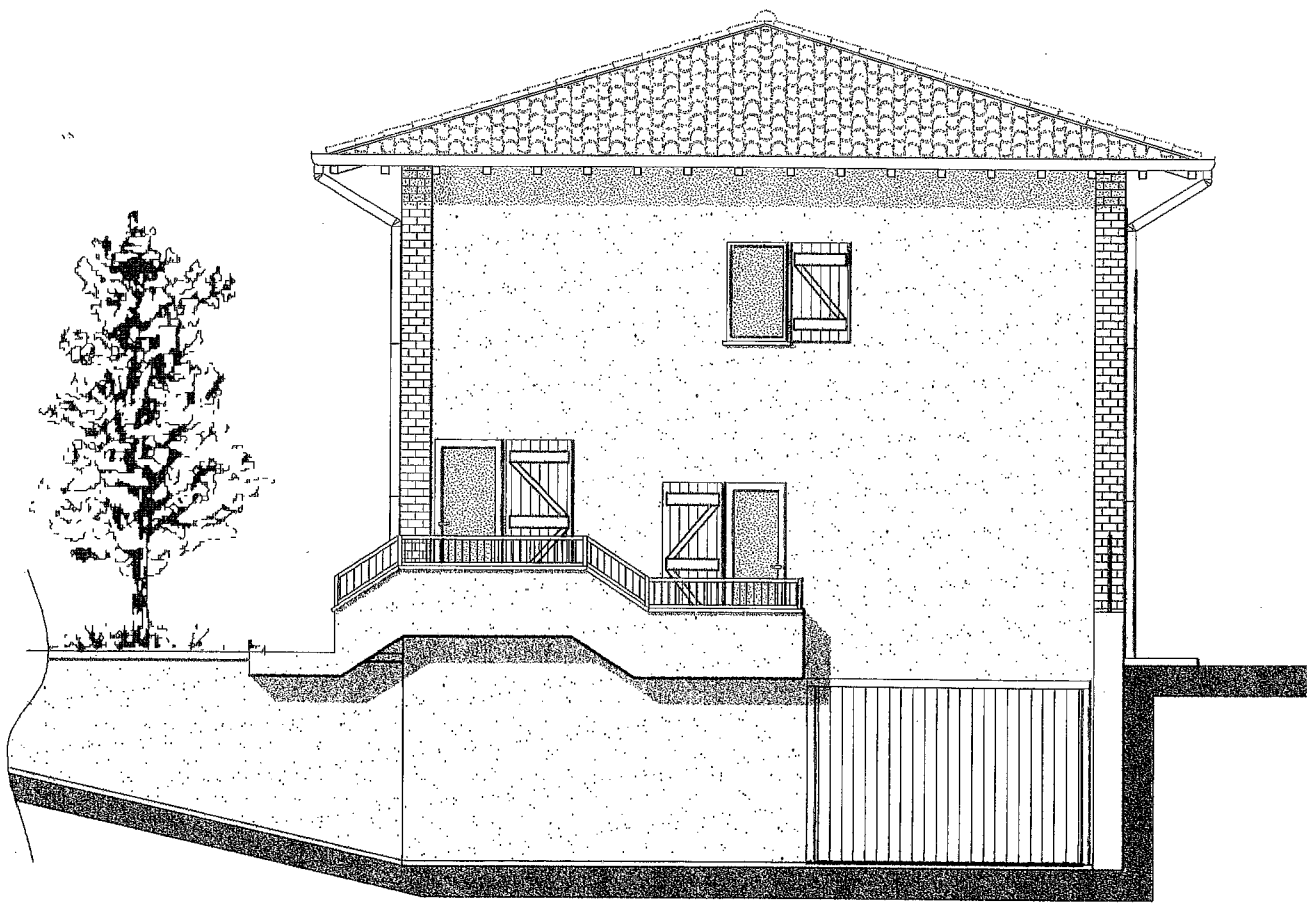
PROSPETTO EST 1:100
